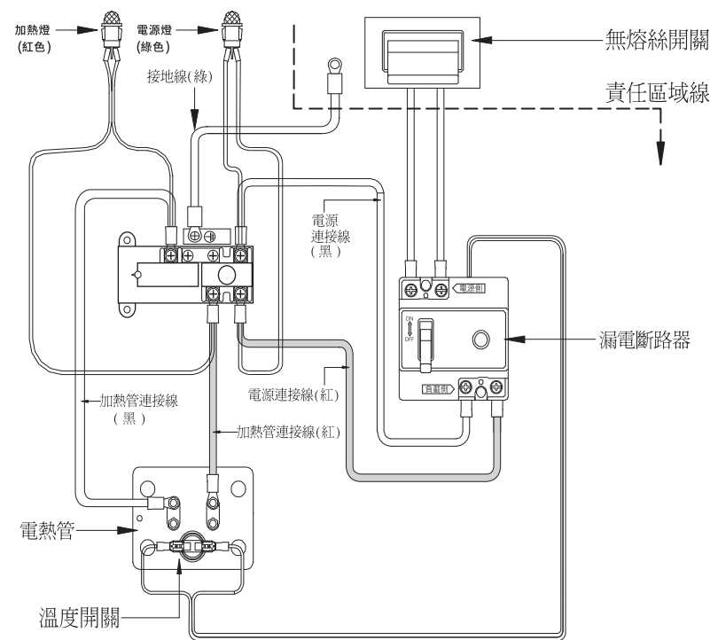
機械式配線圖
