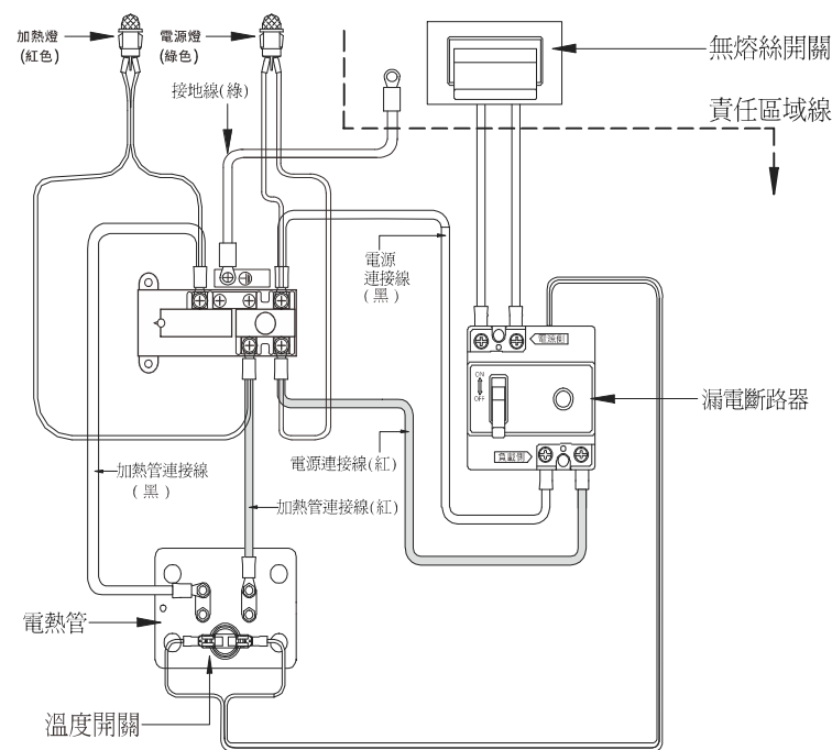
機械式配線圖
